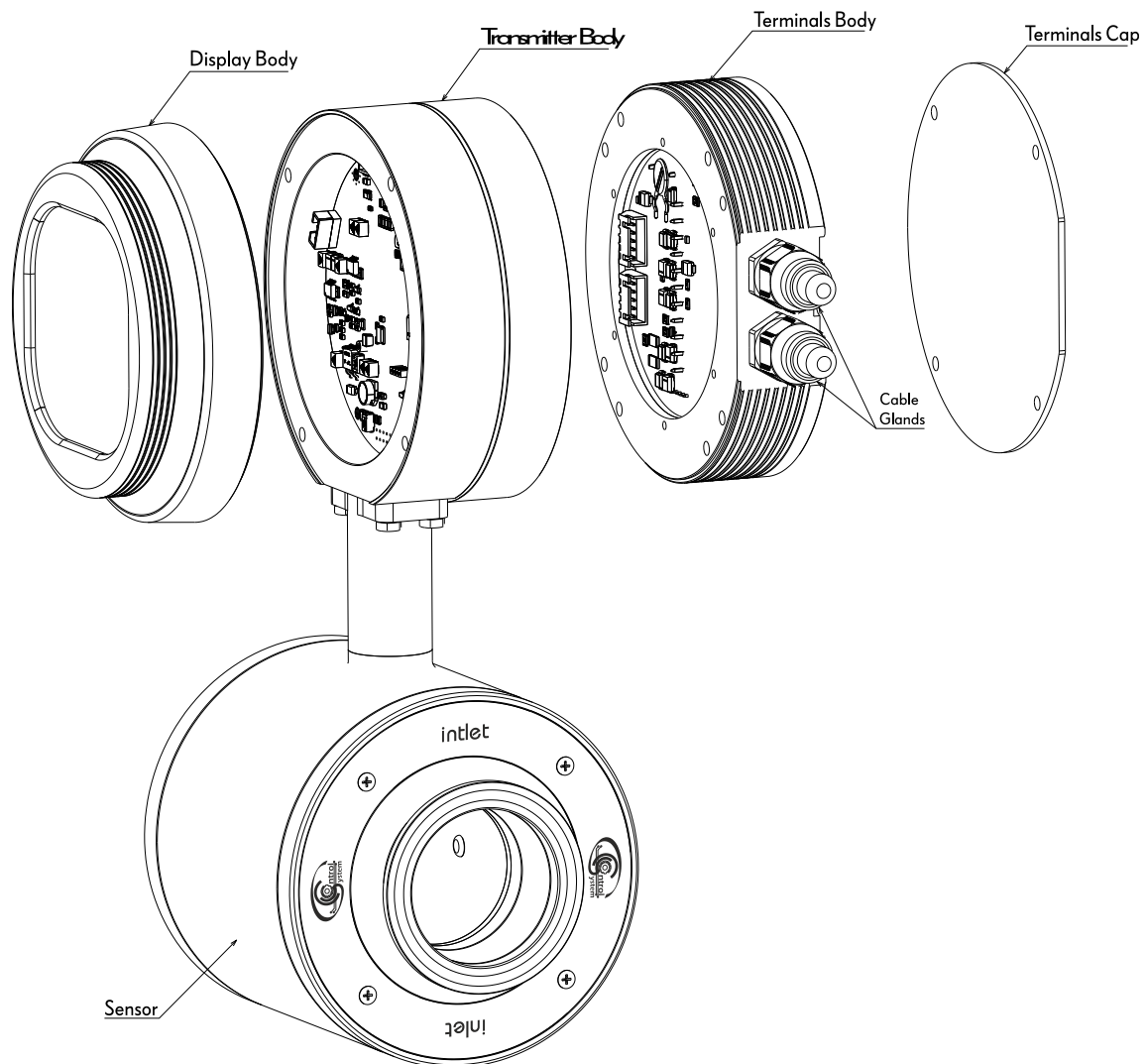
شکل 2-2 بخش‌های مختلف فلومترهای الکترومغناطیسی پریسماتک مدل PTMag
